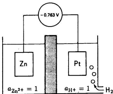
Fig. 25. Determinació del potencial estàndard d'elèctrode.
