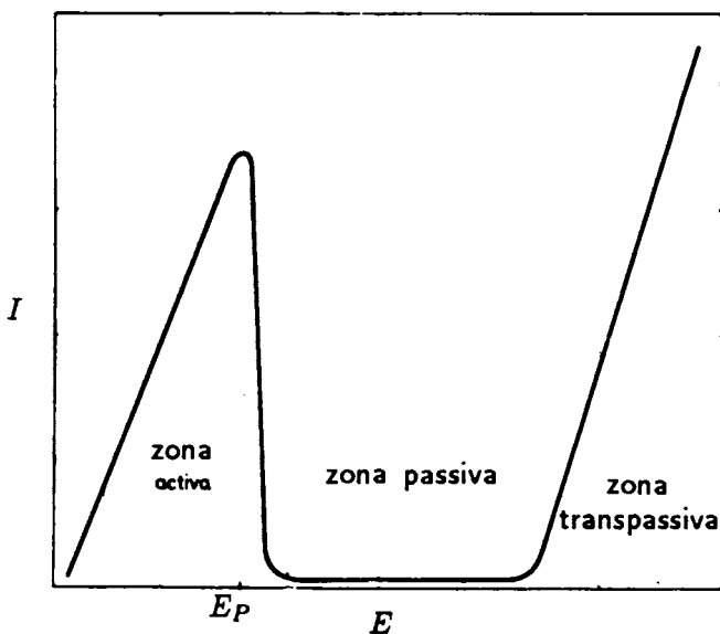
Fig. 28. Corba de polarització anòdica.
