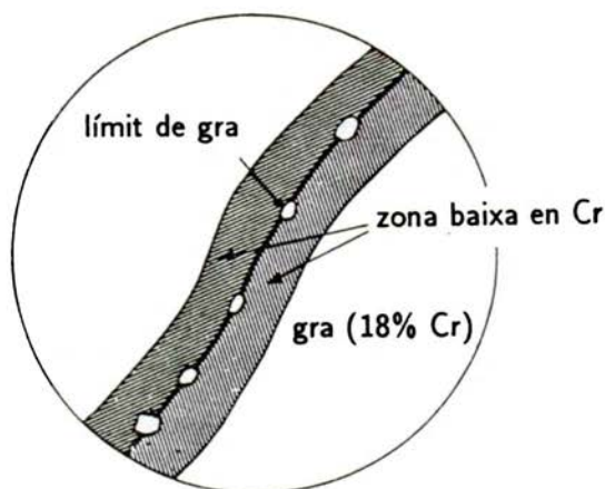
Fig. 21. Límit de gra en un acer inoxidable.
