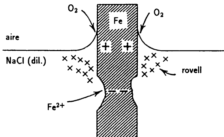
Fig. 22. Pila d'airejament diferencial amb corrosió a la línia d'aigua.
