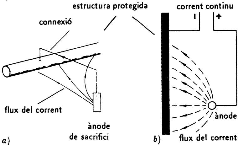
Fig. 26. Protecció catòdica mitjançant: a) ànodes de sacrifici i b) corrent imposat.
