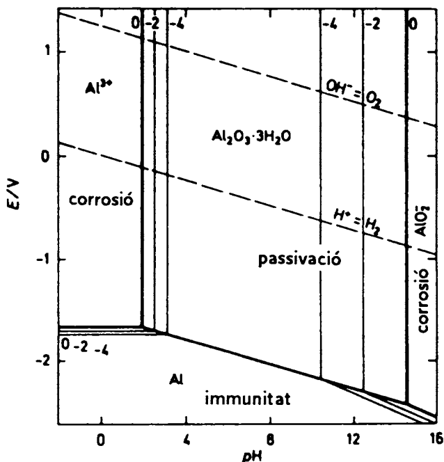
Fig. 13. Diagrama de Pourbaix del sistema alumini-aigua a 25 °C.
