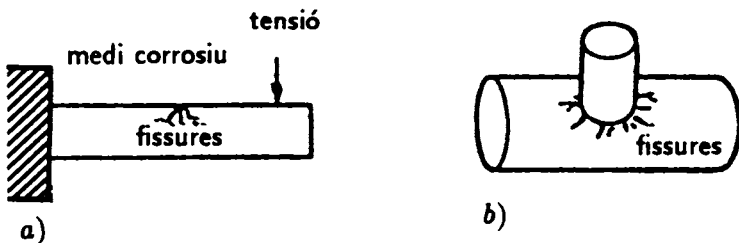
Fig. 11. Model de corrosió sota tensions: a) fissures per tensions i b) fissures per tensions residuals de fabricació.
