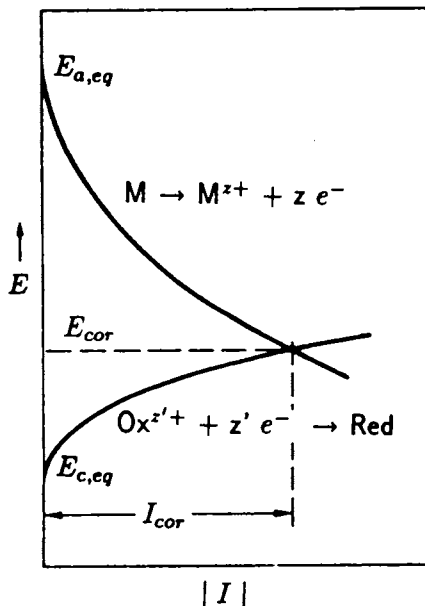
Fig. 12. Diagrama d'Evans simplificat.
