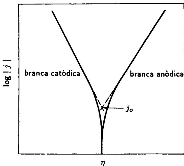
Fig. 14. Diagrama de Tafel simplificat.
