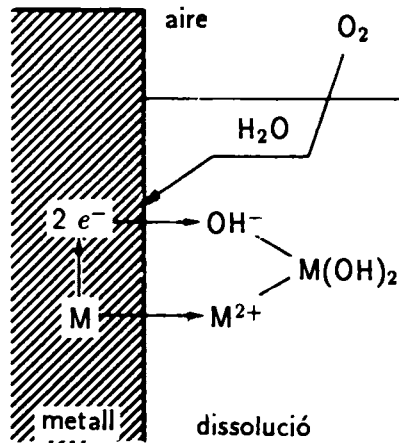
Fig. 5. Model simplificat de corrosió electroquímica.
