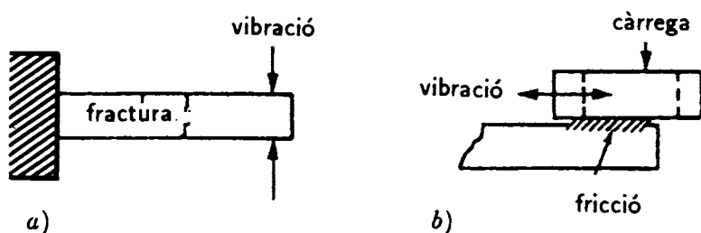
Fig. 6. Models simplificats d'a) corrosió-fatiga i b) corrosió-fricció.
