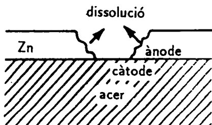
Fig. 20. Acer galvanitzat. El revestiment de zinc es corroeix i, per tant, protegeix el ferro.
