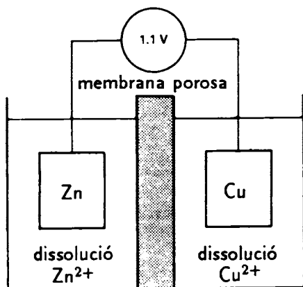
Fig. 23. Esquema d'una pila galvànica.
