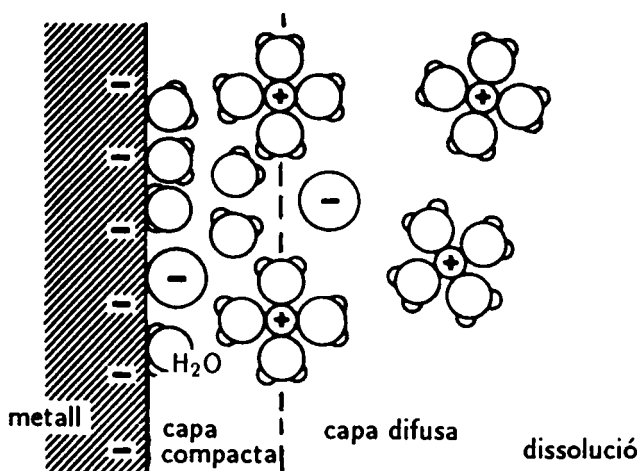
Fig. 15. Model de la doble capa electroquímica.
