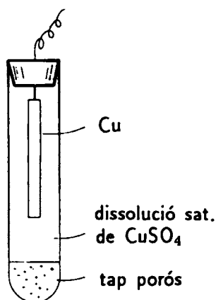
Fig. 17. Elèctrode de referència de \text{CuSO}_4 | Cu.
