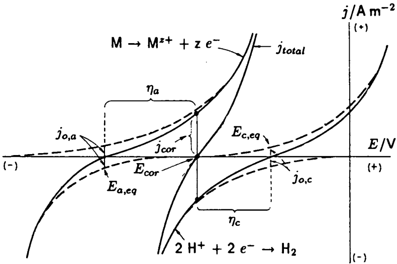
Fig. 3. Corbes de polarització de la reacció dissolució/deposició d'un metall i la reacció redox que l'acompanya.
