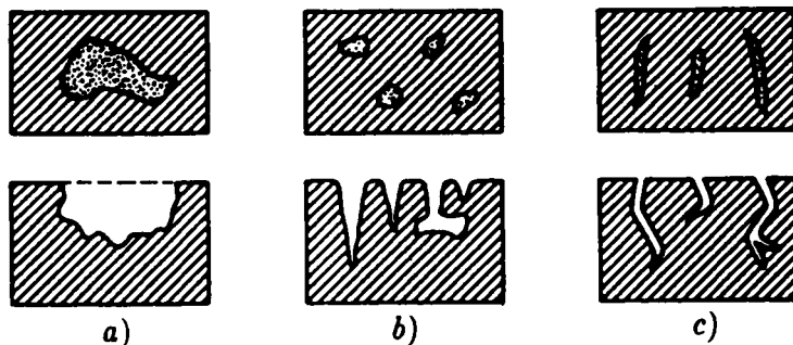
Fig. 9. Formes de corrosió localitzada: a) cràter, b) picadura i c) fissura.
