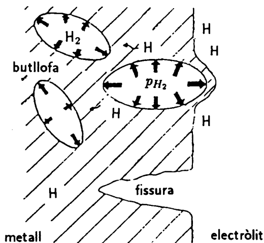
Fig. 18. Model d'embutlofament per hidrogen.
