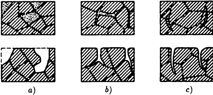
Fig. 10. Formes de corrosió selectiva: a) granular, b) intergranular i c) transgranular.
