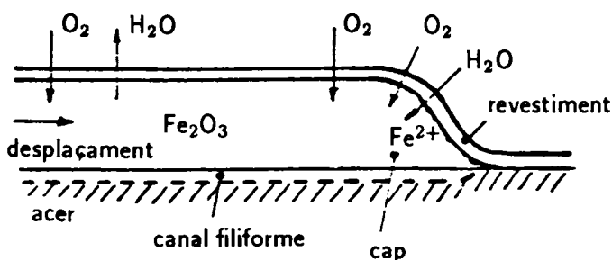
Fig. 7. Secció longitudinal del model de corrosió filiforme.
