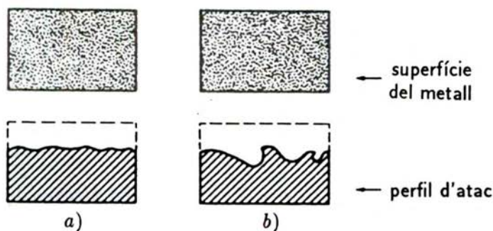
Fig. 8. Formes de corrosió general: a) uniforme i b) irregular.
