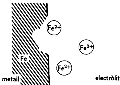
Fig. 1. Ànode de ferro, on el metall es corroeix donant ions ferro.
