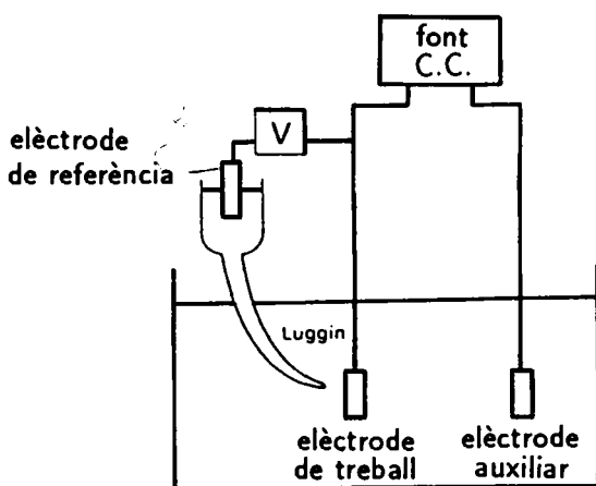
Fig. 16. Sistema de tres elèctrodes per mesurar potencials d'elèctrode.
