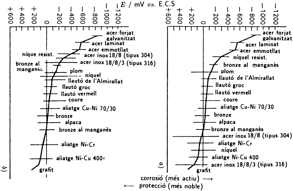
Fig. 27. Sèrie galvànica de metalls i aliatges en: a) aigua de mar airejada i b) aigua desairejada.
